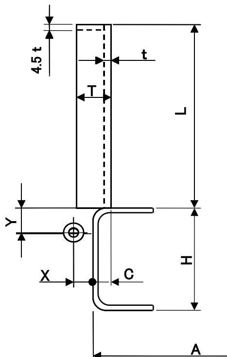
逆蝶番タイプ
